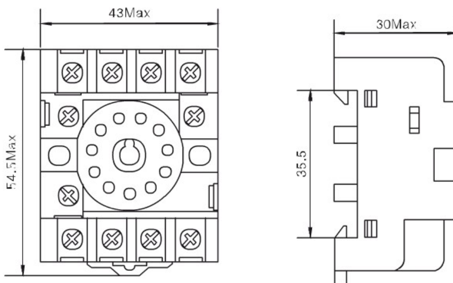
Габаритный чертеж
